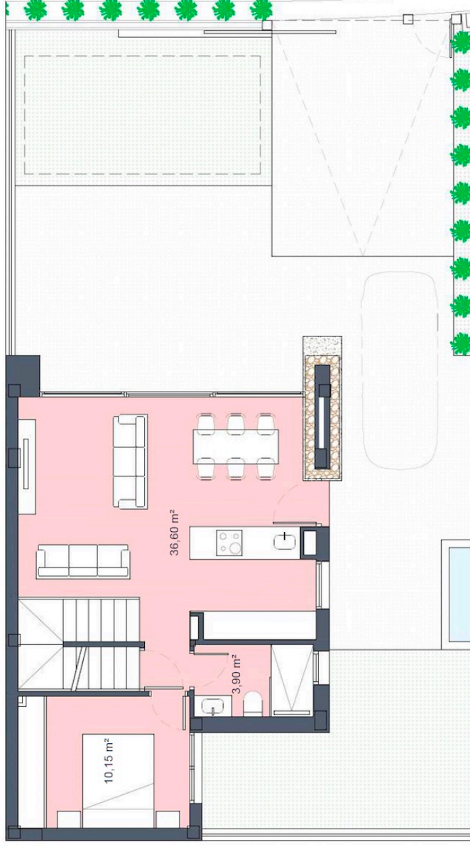
PLANTA BAJA
