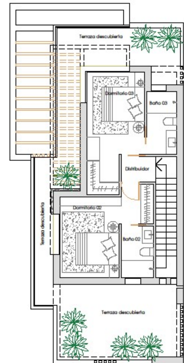
PLANTA PRIMERA
