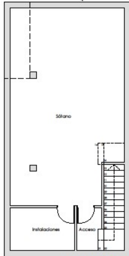
PLANTA SÓTANO
