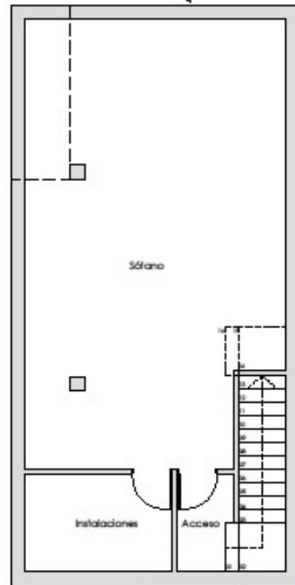
PLANTA SÓTANO
