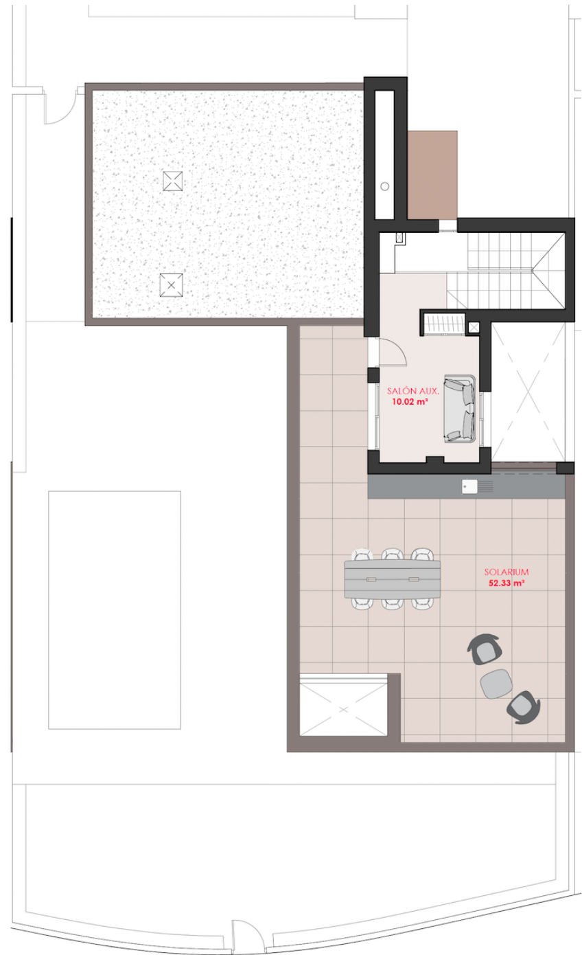
P53.2.1 VIVIENDA 1 PLANTA PRIMERA
